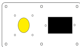
5561/5261 → 1x 16A - 3 polos - salida ángulo IP44 / IP67 - Mennekes: 1463, 1475 . // 1x IP55 - hasta 4 mód. - cód. 6993 , tapa y bastidor para intemperie.
