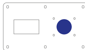
5562/5262 → Espacio para térmicas // 1x 16A - 3, 4, 5 polos - salida recta IP44 / IP67 - Mennekes: 1366, 1390, 1385, 218, 222, 228 // ó // 1x 32A - 3, 4, 5 polos - salida recta IP44 / IP67 - Mennekes: 1395, 1399, 3451, 230, 234, 240 .
