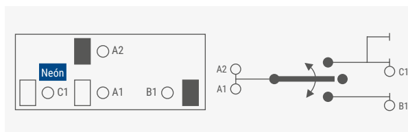
Esquema 5: Interruptor para persianas 9535/7535.
