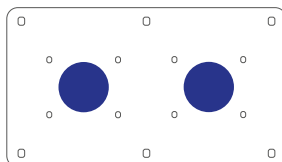
5552/5252 → 16A - 3, 4, 5 polos - salida recta IP44/IP67 - Mennekes: 1366, 1390, 1385, 218, 222, 228 . // o // 32A - 3, 4, 5 polos - salida recta IP44/IP67 - Mennekes: 1395, 1399, 3451, 230, 234, 240 .
