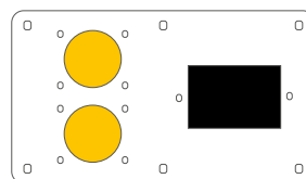
5557/5257 → 2x 16A - 3 polos - salida recta IP44 Schuko 10436 // 1x IP55 - hasta 4 mód. - cód. 6993 , tapa y bastidor para intemperie.
