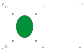
5556/5256 → 1x 16A - 4, 5 polos - salida ángulo IP44 / IP67 - Mennekes: 1467, 1473, 1479, 1485 // o // 1x 32A - 3, 4, 5 polos - salida ángulo IP44 / IP67 - Mennekes: 1492, 1496, 1500, 1502, 1506, 1551 .
