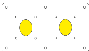
5555/5255 → 2 x 16A - 3 polos - salida ángulo IP44 / IP67 - Mennekes: 1463, 1475 .
