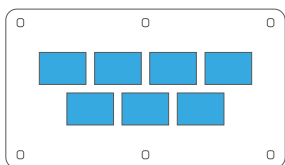
5559/5259 → 7 espacios para tomas Cambre // 10A - 1, 2 mód. - cód: 6911, 6903, 6904, 6909, 6912 // 16A - 2 mód. - cód: 6917, 6918 // 20A - 2 mód. - cód. 6915 .
