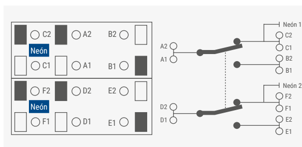
Esquema 4: Interruptor para persianas 9534/7534.
