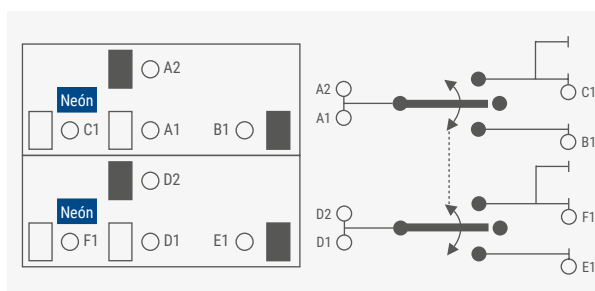
Esquema 5: Interruptor para persianas 9535/7535.
